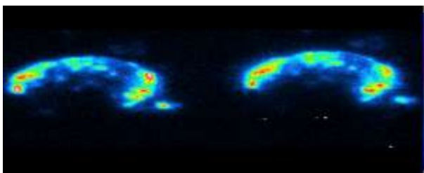
Th 227 (α線) で標識された腫瘍サンプル
